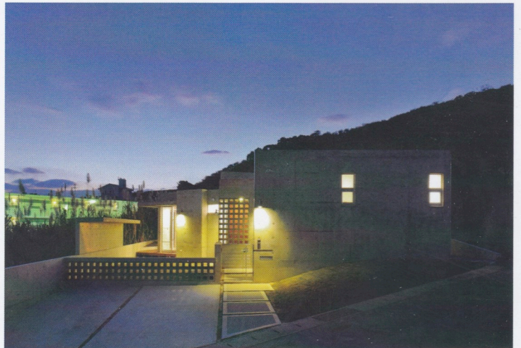
右の外観写真からもわかるように、高低差のある土地に設計したこの家は、外壁も内壁コンクリート打ちっばなしにしたモダンな設計。室内はスキップフロアにしていることから、平屋でありながら暮らしにリズムが生まれる。コンクリートの台座にステンレスの天板を持つカウンターキッチンと無垢材のキッチンボードは造作。シンプルでありながら、高いデザイン性を併せ持つ空間にまとめられている
